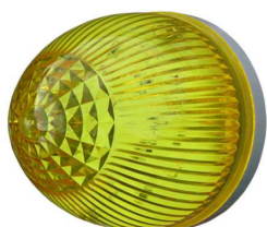
LEDマーカー 2561Y 部品コード：4HA165 灯体寸法 85φ×75mm 定格入力電圧 24V 定格消費電力 1.65W
