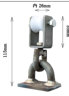
トリプルシャックル（30φ シープ付） 部品コード：2SI072
