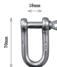
9mm 長シャックル 部品コード：2SI059
