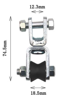
ターン・シャックル S-B 部品コード：2SI066
