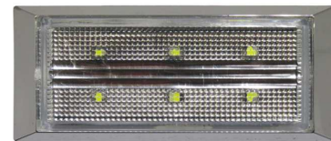
ポイントマーカー CE-147 C/W 部品コード: 2YGHHS 灯体寸法 (mm) 95(W)×45(H)×10(D) 定格入力電圧 DC12V、DC24V
