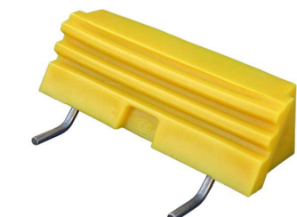
ハイプラ輪止め（ピン幅 200mm） 高さ：90mm 部品コード：2HH053
