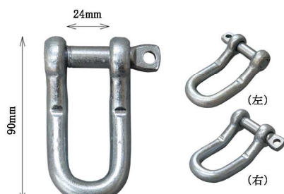
12mm 長シャックル（曲げ加工） 部品コード：2SI052（左） 部品コード：2SI053（右）
