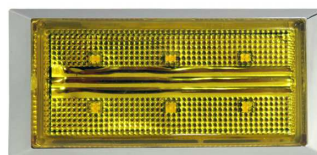
ポイントマーカー CE-141Y 部品コード: 2YGHY 灯体寸法 (mm) 95(W)×45(H)×10(D) 定格入力電圧 DC12V、DC24V
