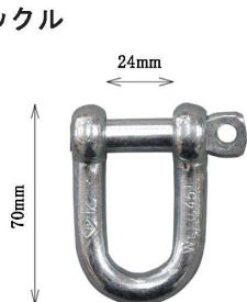
12mm シャックル 部品コード：2SI060
