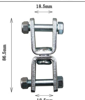
ターン・シャックル M（枠のみ） 部品コード：2SI083
