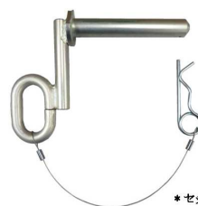
ローダウン・ピン (ワイヤ、Rピン付)
