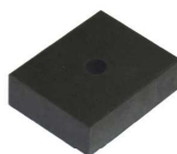
サイレンサー (ゴム製、1 穴) 15t×40mm×50mm 部品コード：7TG004
